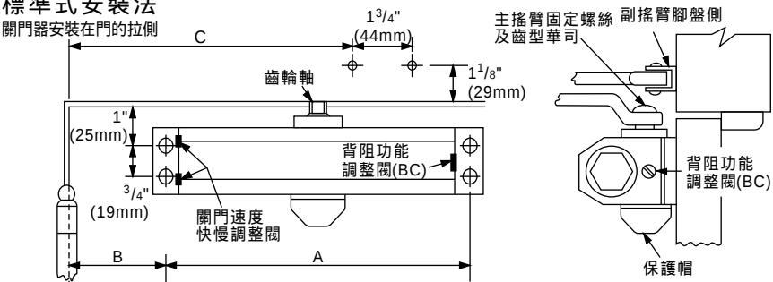
右開門安裝示意圖 安裝尺寸應用表（左開門時亦同）
